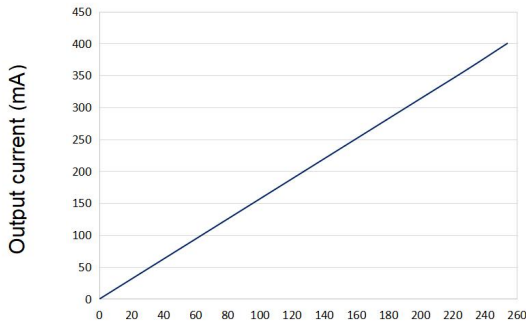
Linear dimming
